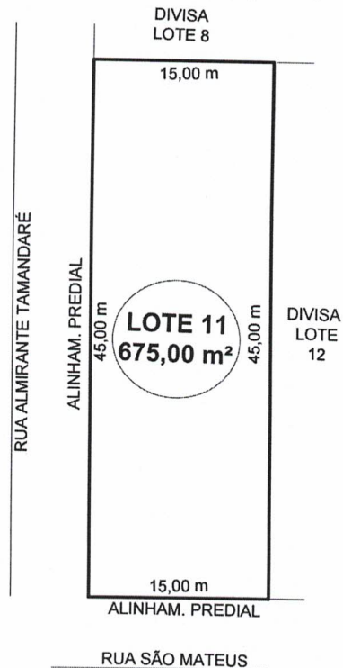
PLANTA DO LOTE ESCALA: 1:750
