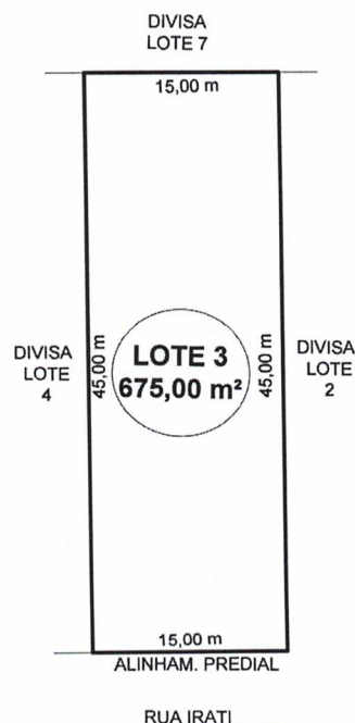
PLANTA DO LOTE ESCALA: 1:750
