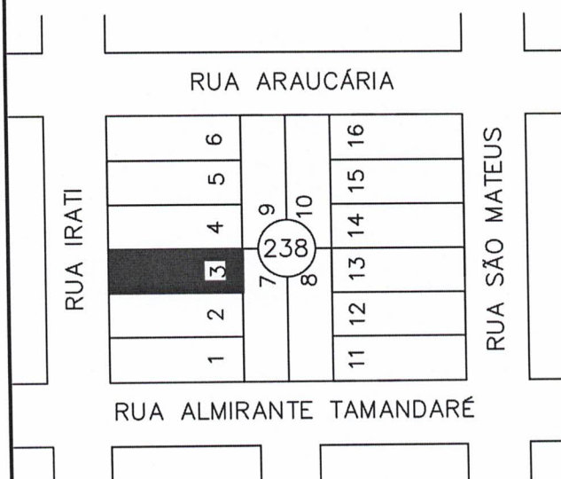
PLANTA DE SITUAÇÃO ESCALA: 1:2000
